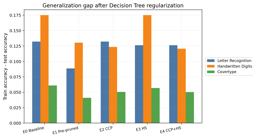
Hình 5.2: Train-test gap của các cấu hình cải tiến trên ba bộ dữ liệu.
